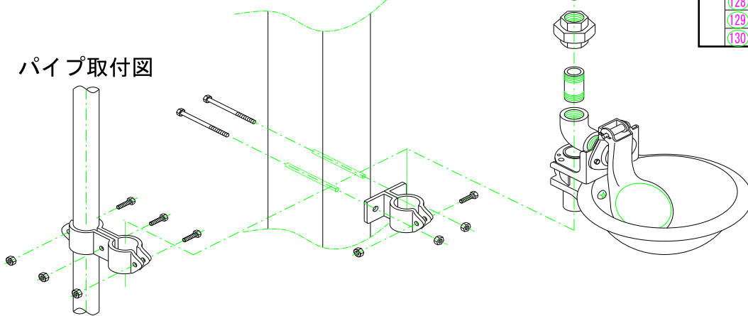
木柱取付図
