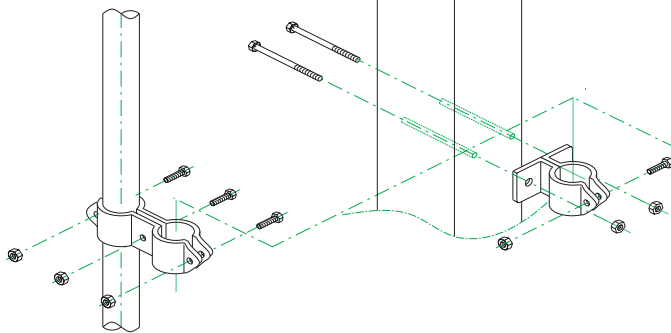
パイプ取付図
