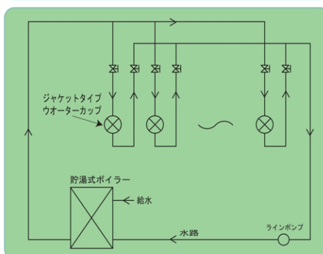
システム・フロー図
